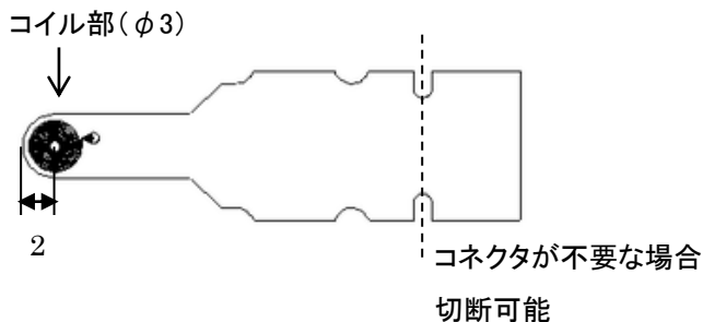
<部品実装面>
