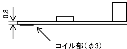
<コイル仕様>
